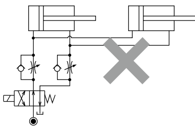
【Meter-in Circuit】
